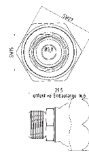
RE-2-G1/4 Reduktion Typ 2 auf G 1/4" reduction Type 2 to G 1/4"
