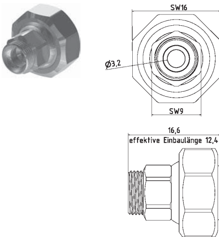
RE-1-0 Reduktion Typ 1 auf Typ 0 reduction Type 1 to Type 0
