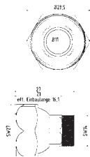
RE-2-1 Reduktion Typ 2 auf Typ 1 reduction Type 2 to Type 1
