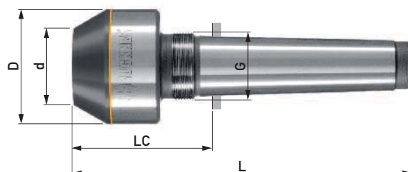
Form GR großer Hartmetallring bis \varnothing 100 mm
