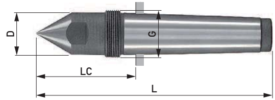
Form 255 ähnlich DIN 807 und verlängert
